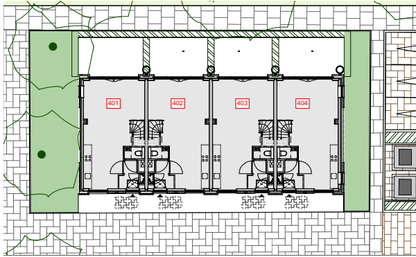
begane grond Gebouw 4 (OVERZICHT) schaal 1 : 100
