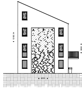
Zuidgevel schaal 1:100
