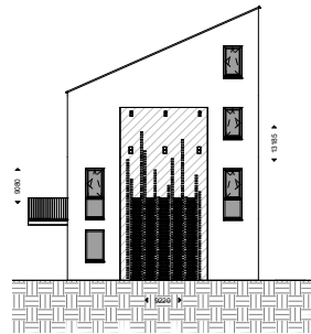
Noordgevel schaal 1:100
